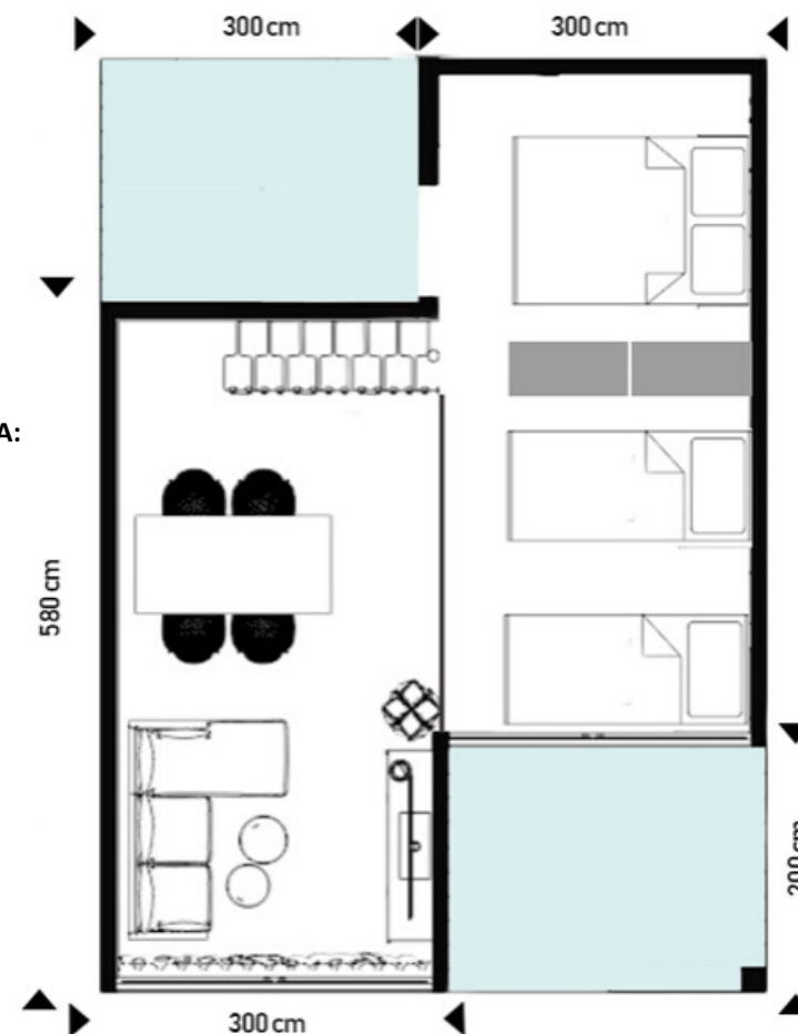
RZUT PIĘTRA
